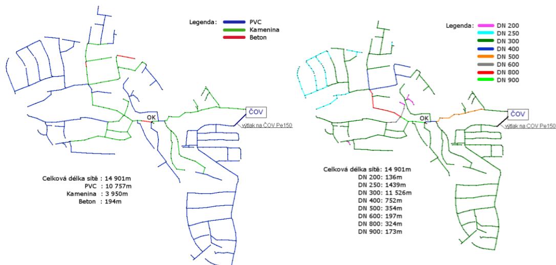
Obr.2. Materiálová skladba a profily stokové sítě.
